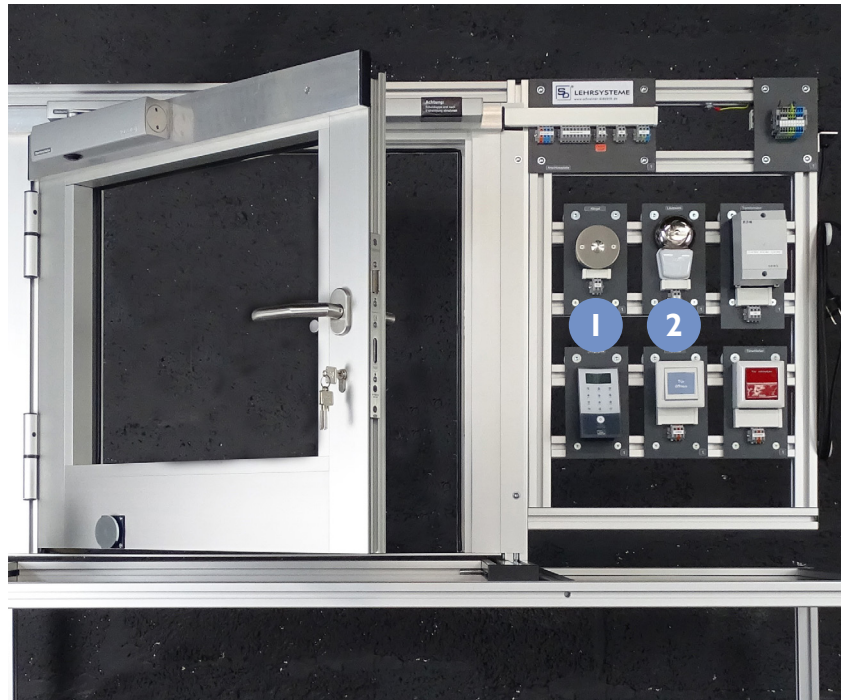
Abbildung zeigt: 144954 –Tischmodell Aluminiumtür und Montagefeld 144954.2, Modulsatz elektrischer Türöffner 144954.3, Modulsatz Feststelanlage mit Rauchmelder 144954.5, Fingerprint 144954.10, Ergänzungssatz Klingelplatte mit Klingel 144954.3.1, Haftmagnet 144954.9
